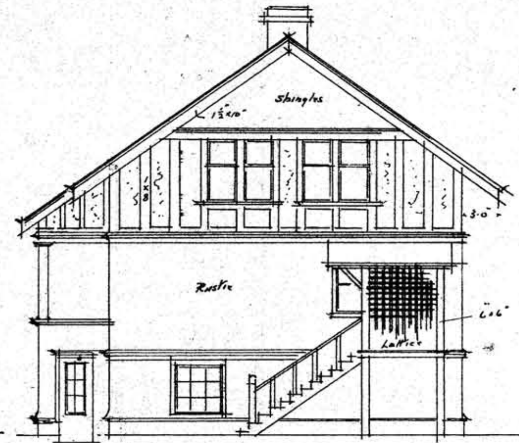
END ELEVATION
